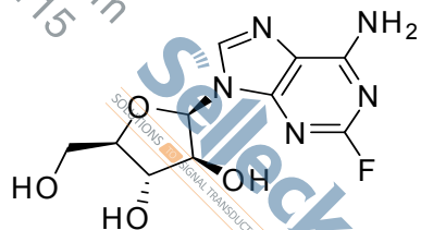
S149101, DMSO-d6
