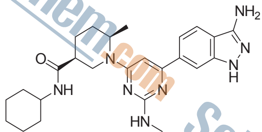
S708702, DMSO-d6
