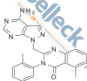
S220701, DMSO-d6
