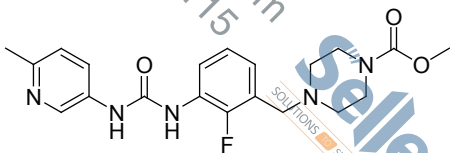
S262301, DMSO-d6
